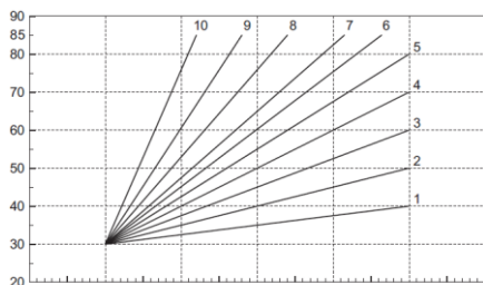
rys. 6 - Krzywe kompensacji
