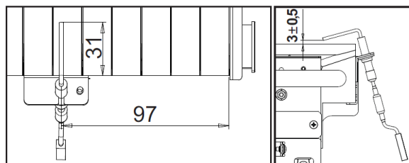
rys. 14 - Pozycjonowanie elektrody
