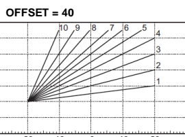
rys. 7 - Przykład przesunięcia równoległego krzywych kompensacji
