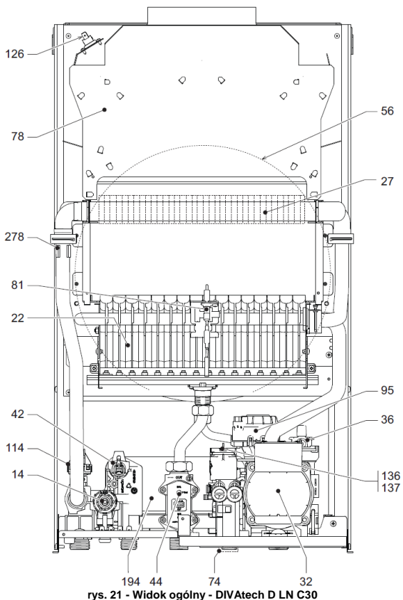
rys. 21 - Widok ogólny - DIVATech D LN C30
