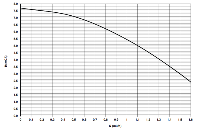
Dostępna resztkowa różnica ciśnień w instalacji DIVATech D LN C30
