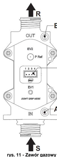
rys. 11 - Zawór gazowy
