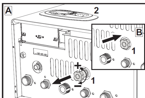
rys. 8 - Pokrętło napełniania
