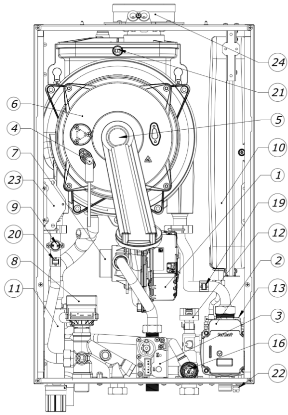
Kocioł jednofunkcyjny
